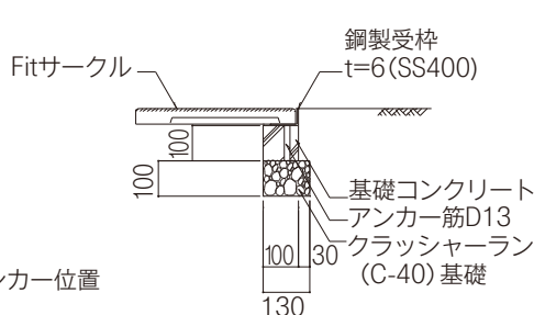
施工断面図
