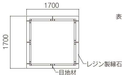
SS/SEタイプ 平面図
