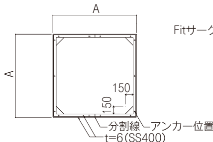
SS/SEタイプ 平面図
