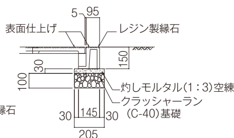
施工断面図
