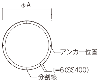
EE/ESタイプ 平面図
