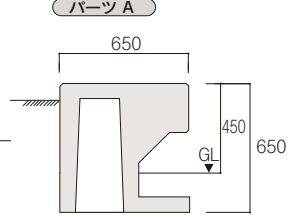
八角形 TB-04
