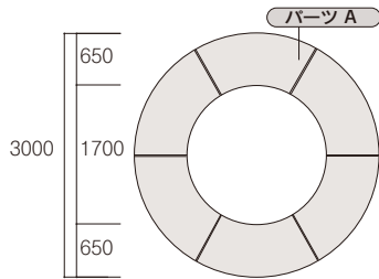
丸形 TB-02
