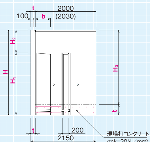
側面図
