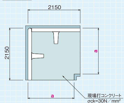
施工平面図
