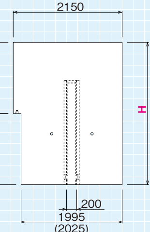
右側部材
