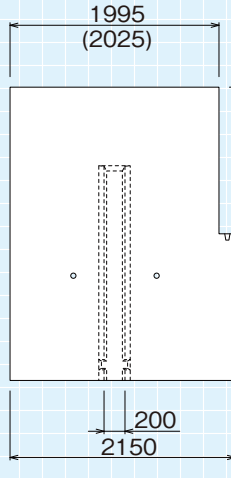
側面図
