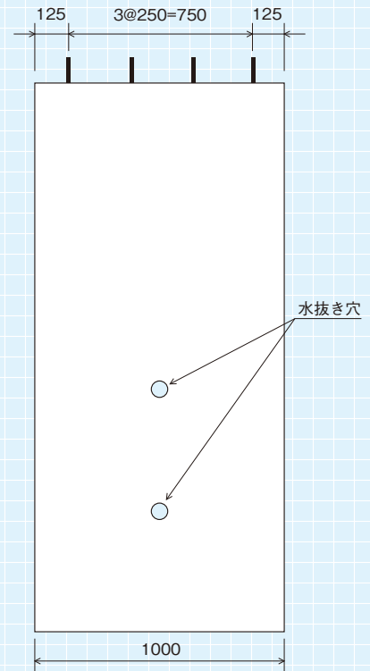
正面図
