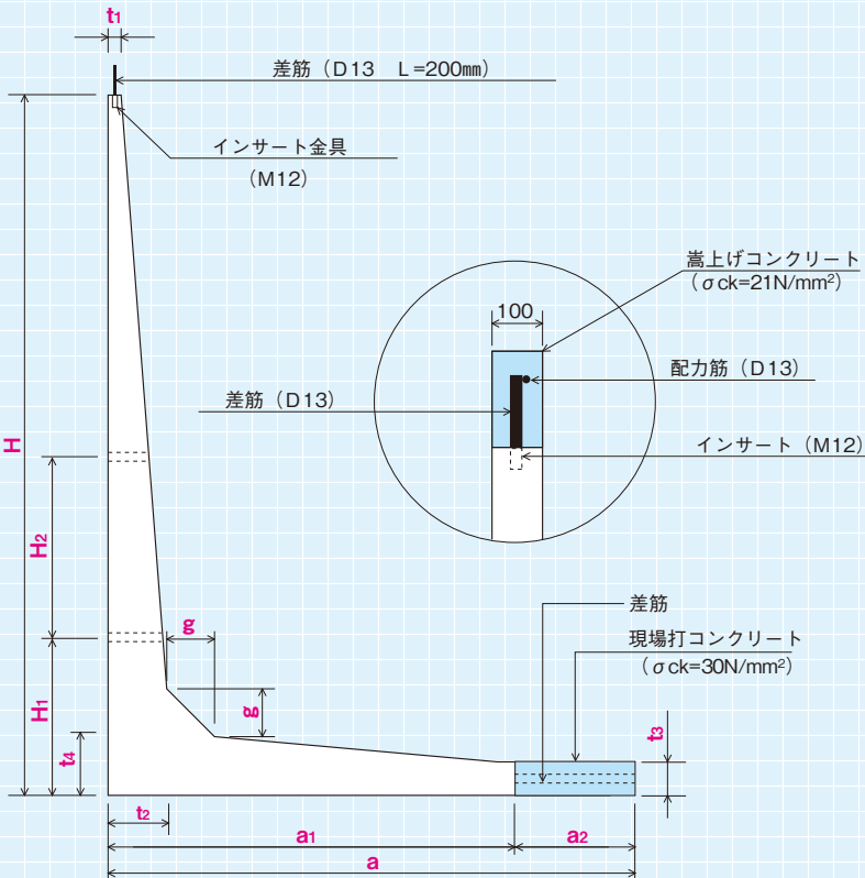
側面図
