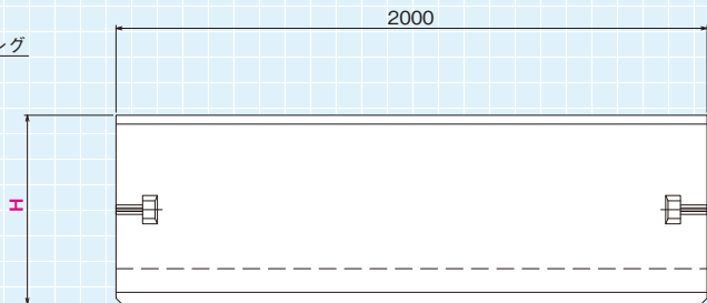
側面図
