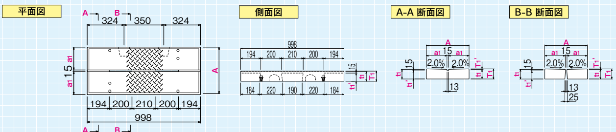
標準蓋 L = 1000
