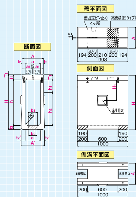
標準 L = 1000
