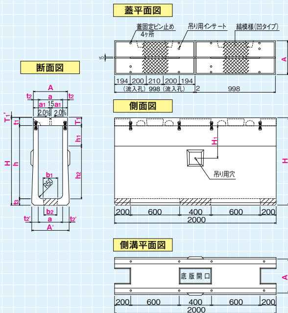
標準蓋 L = 1000
