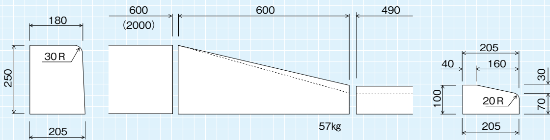
片面歩車道B(基本2種)~FN乗入れ(タイプ2)用1本切下げ
