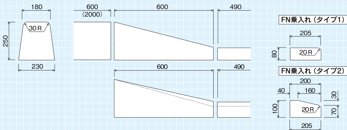
両面歩車道B(180/230×250)~FN乗入れ(タイプ1、2)用1本切下げ
