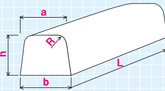
歩車道境界ブロック両面R
