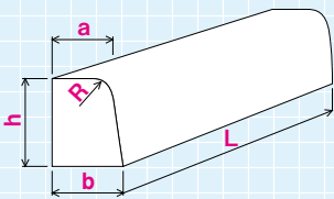
歩車道境界ブロック
