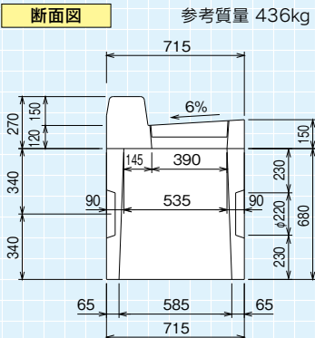
断面図
