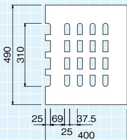
断面図
