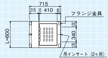
平面図
