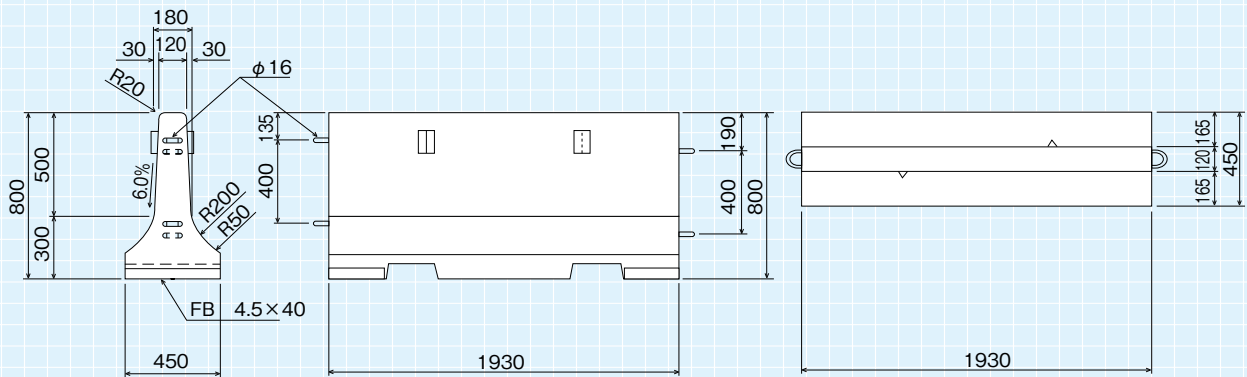
正面図
