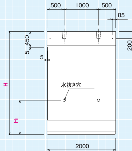
背面図
