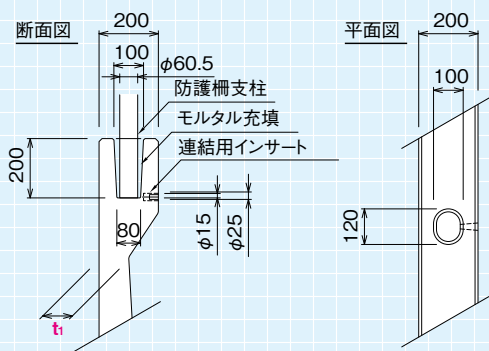
天端形状詳細図
