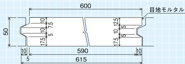
詳細図
