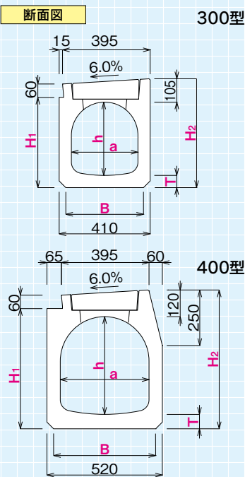
断面図
