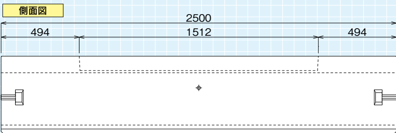
側面図
