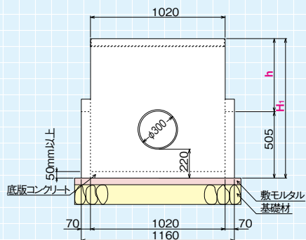
側面図
