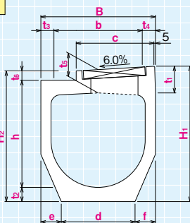
断面図
