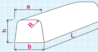
歩車道境界ブロック両面R
