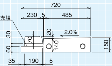
B-B 断面
