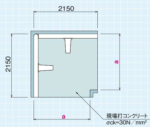
施工平面図
