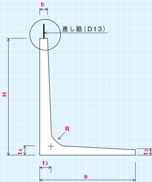
側面図
