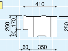
側面図
