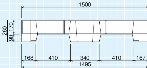
正面図
