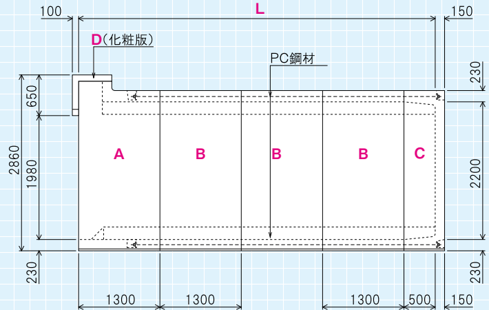
側面図
