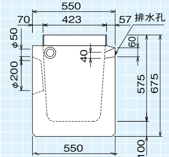
断面図
