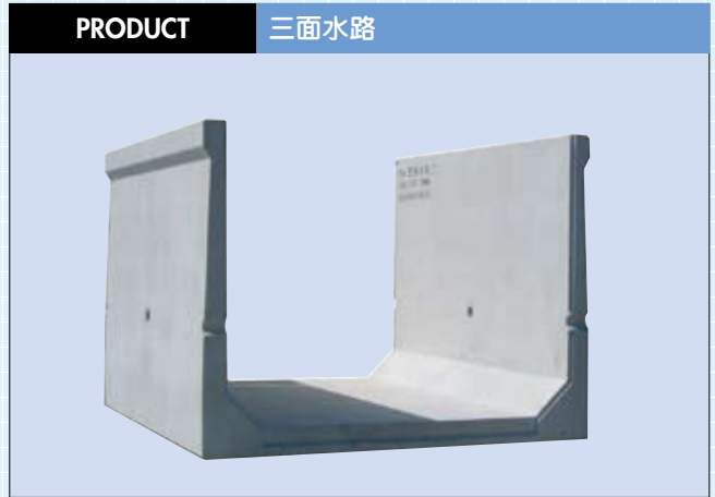
T-25、T-14 は形状・寸法同一で配合・配筋等で調整致します。
