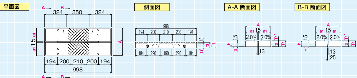
標準蓋 L = 1000
