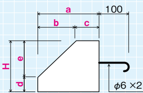
側面図
