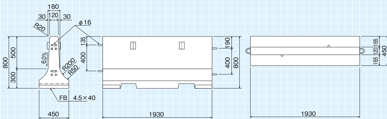
正面図
