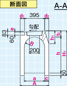
断面図
