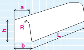
歩車道境界ブロック
