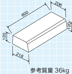
歩道乗入れ部
