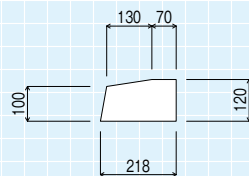
平面図
