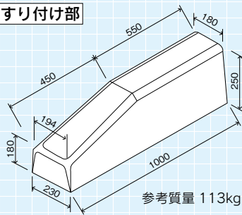
■マウンドアップ型
