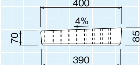
断面図
