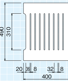
断面図
