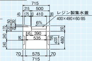
断面図
