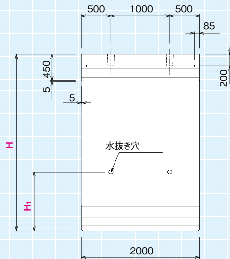
背面図
