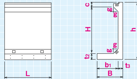
端部L型
