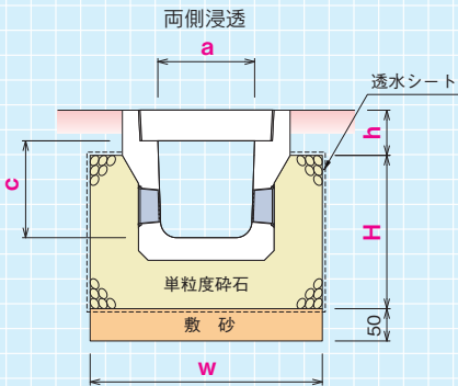
●寸法表 (落蓋側溝)
