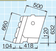
側面図
