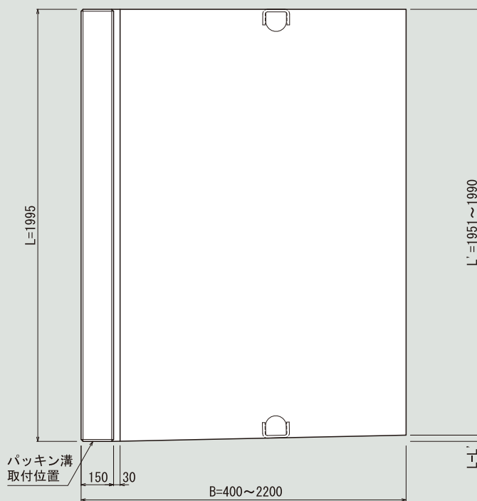
平面図 S=1:10
